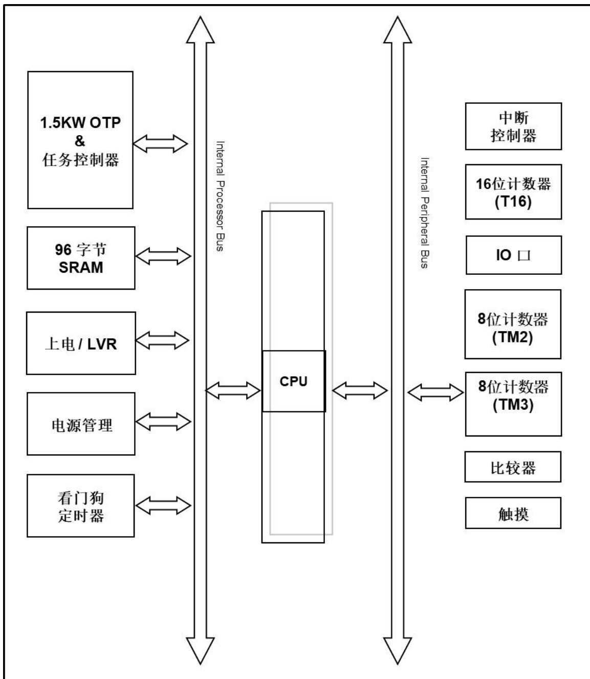
图 1: JZ8P115 系统方框图
