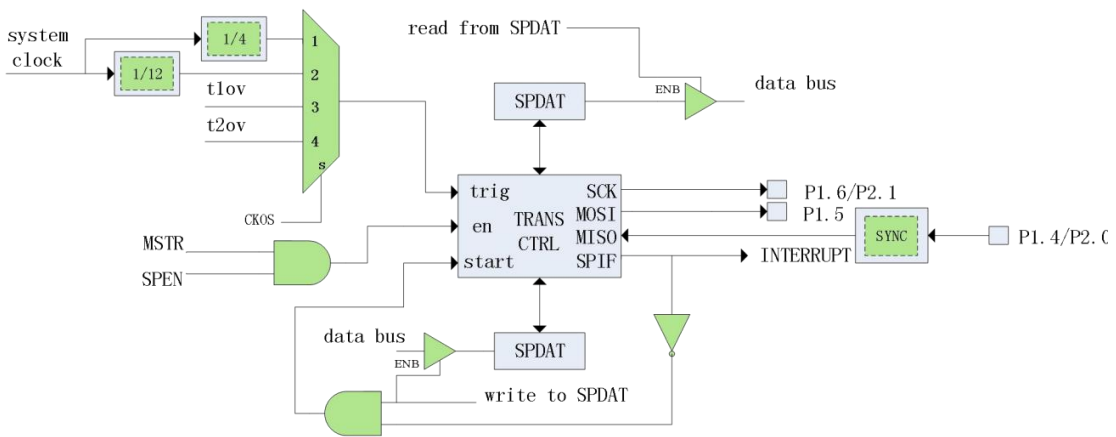
图 19-1-1 SPI 主机模式示意图
