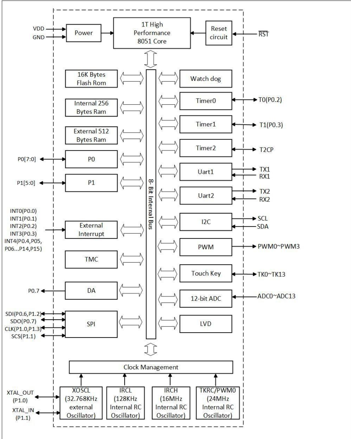
图 4-1-1 芯片框图
