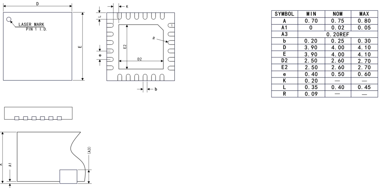
QFN24 封装尺寸
