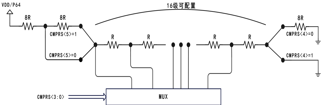
比较器修调示意图
