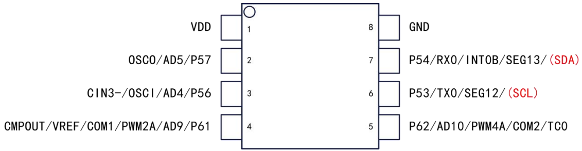
JZ8M4601-8PIN 脚位图
