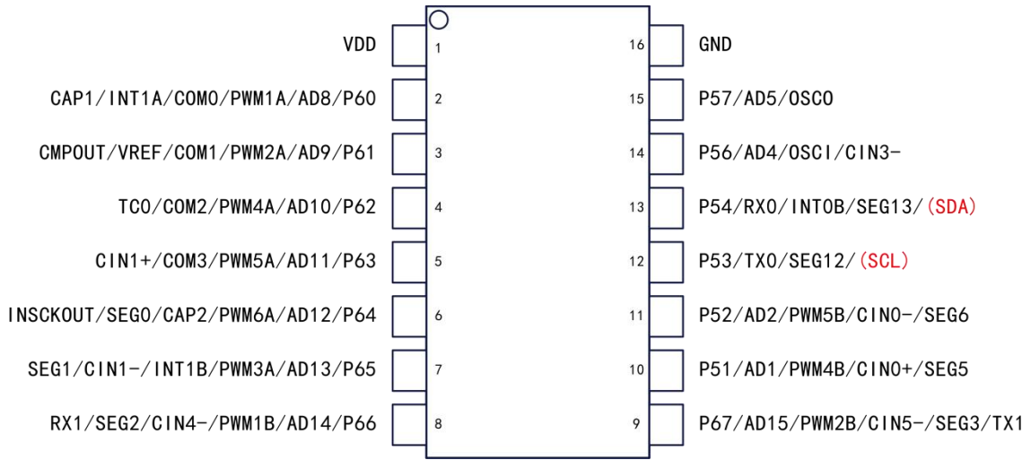
JZ8M4601-SOP16 脚位图
