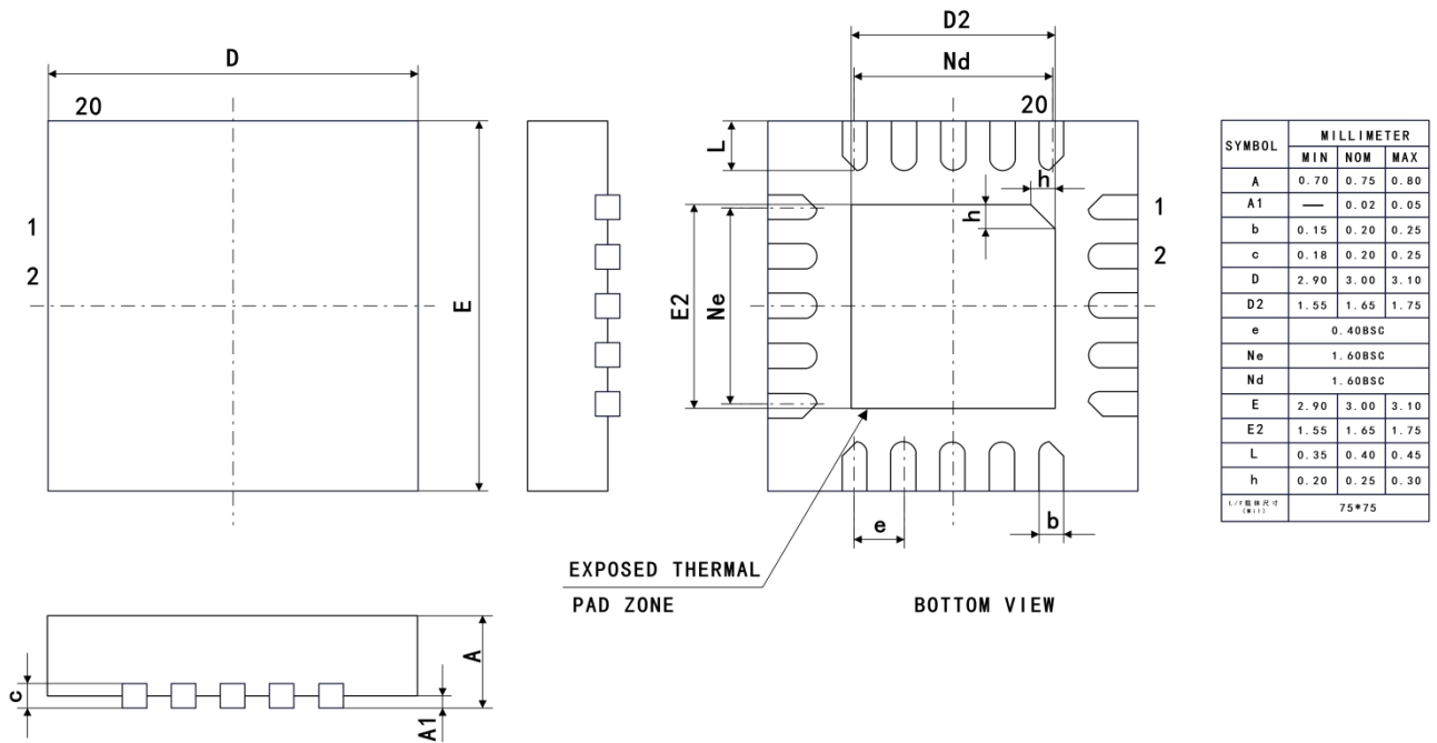
QFN20 封装尺寸
