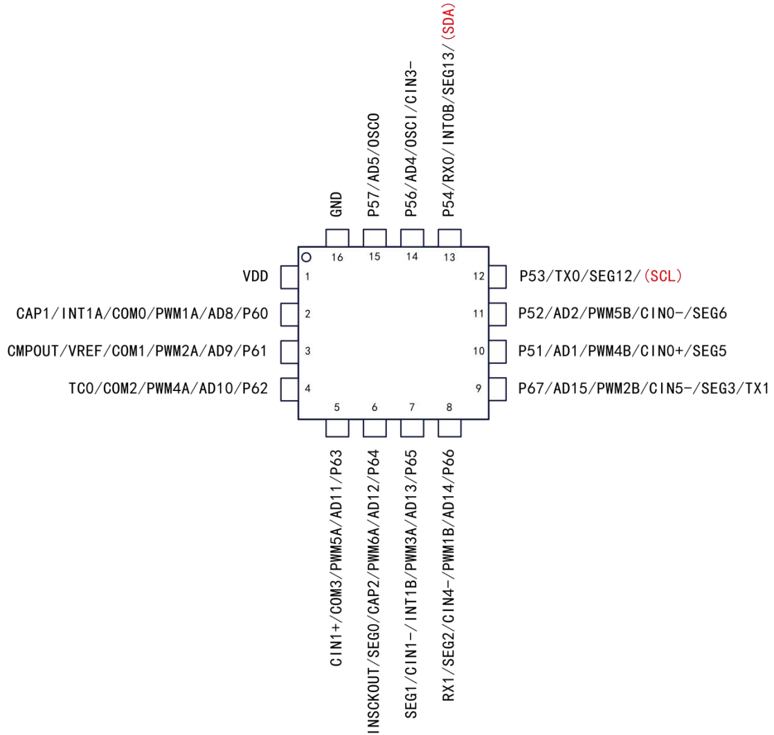
JZ8M4601-QFN16 脚位图
