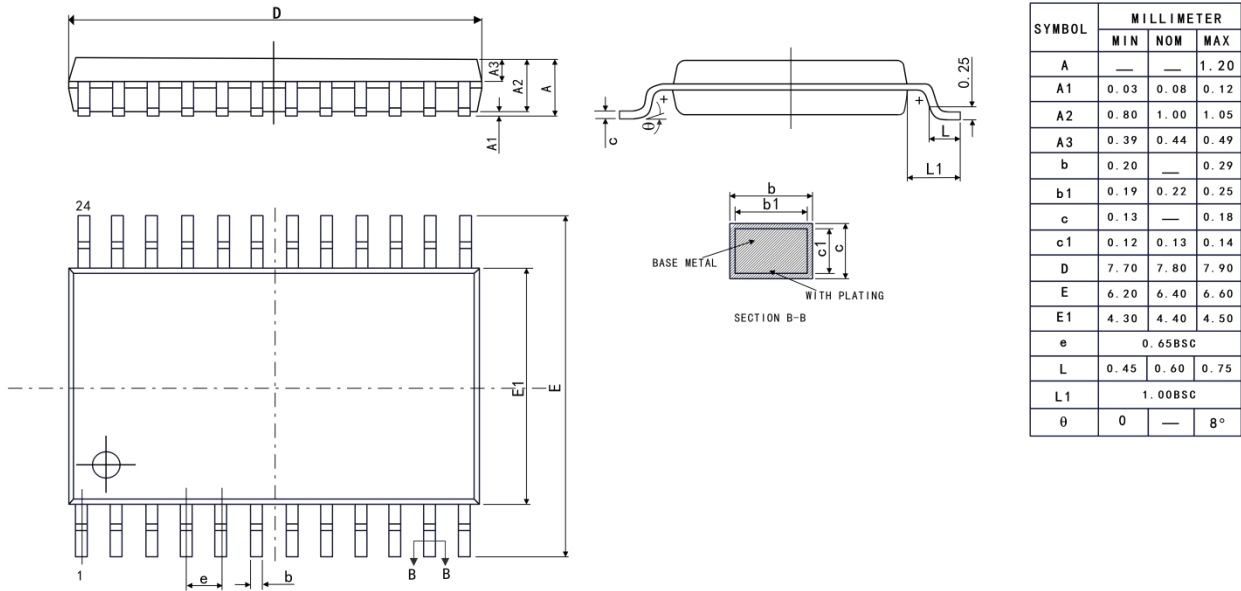
TSSOP24 封装尺寸
