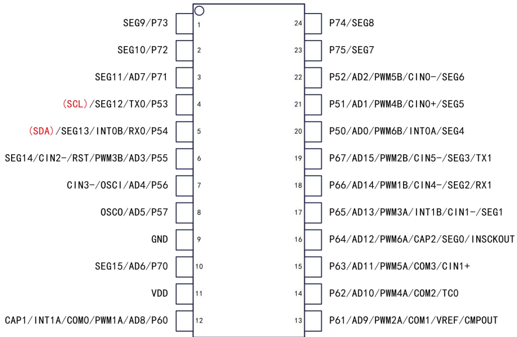
JZ8M4601-TSSOP24 脚位图
