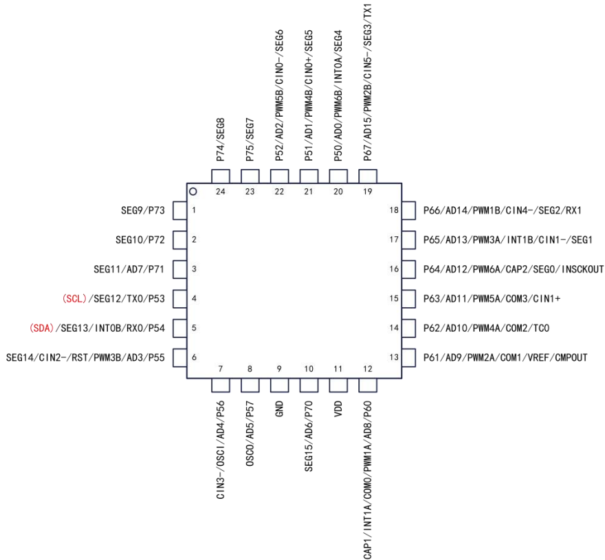
JZ8M4601-QFN24 脚位图
